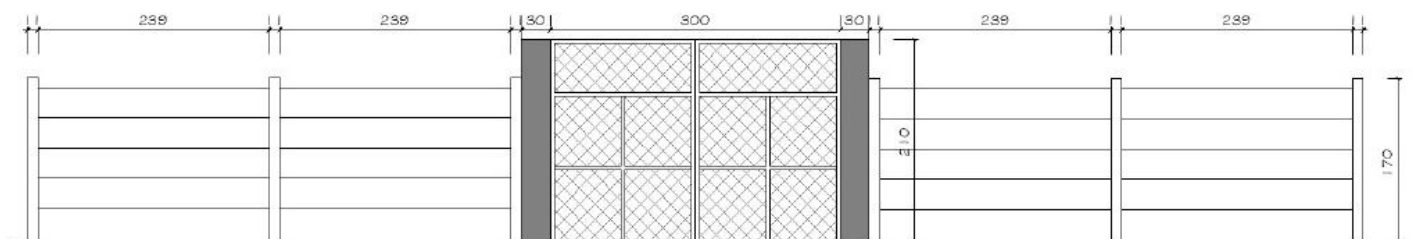
Figura ilustrativa 06 – Fonte: Projeto Arquitetônico (Detalhe gradil)
