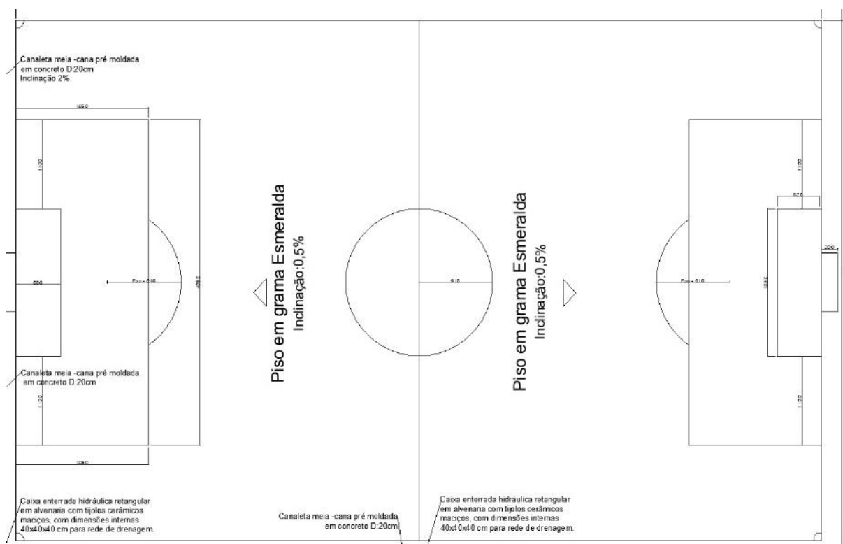
Figura ilustrativa 01 – Fonte: Projeto Arquitetônico
