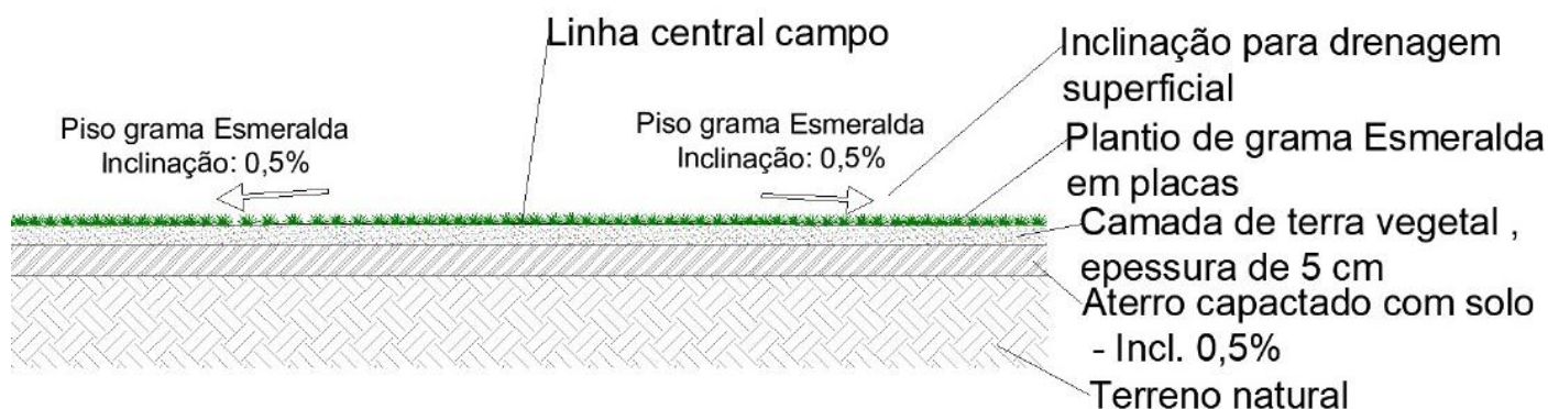
Figura ilustrativa 02 – Fonte: Detalhamento Projeto Arquitetônico
