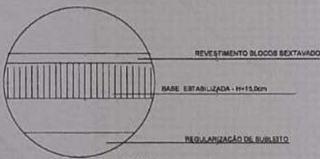
CORTE TIPO
