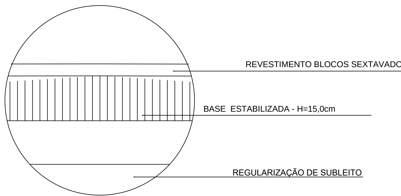
DETALHE 01 S/ESCALA
