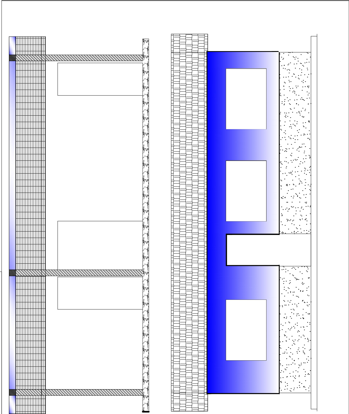
CORTE LONGITUDINAL - BB' FACHADA FRONTAL
