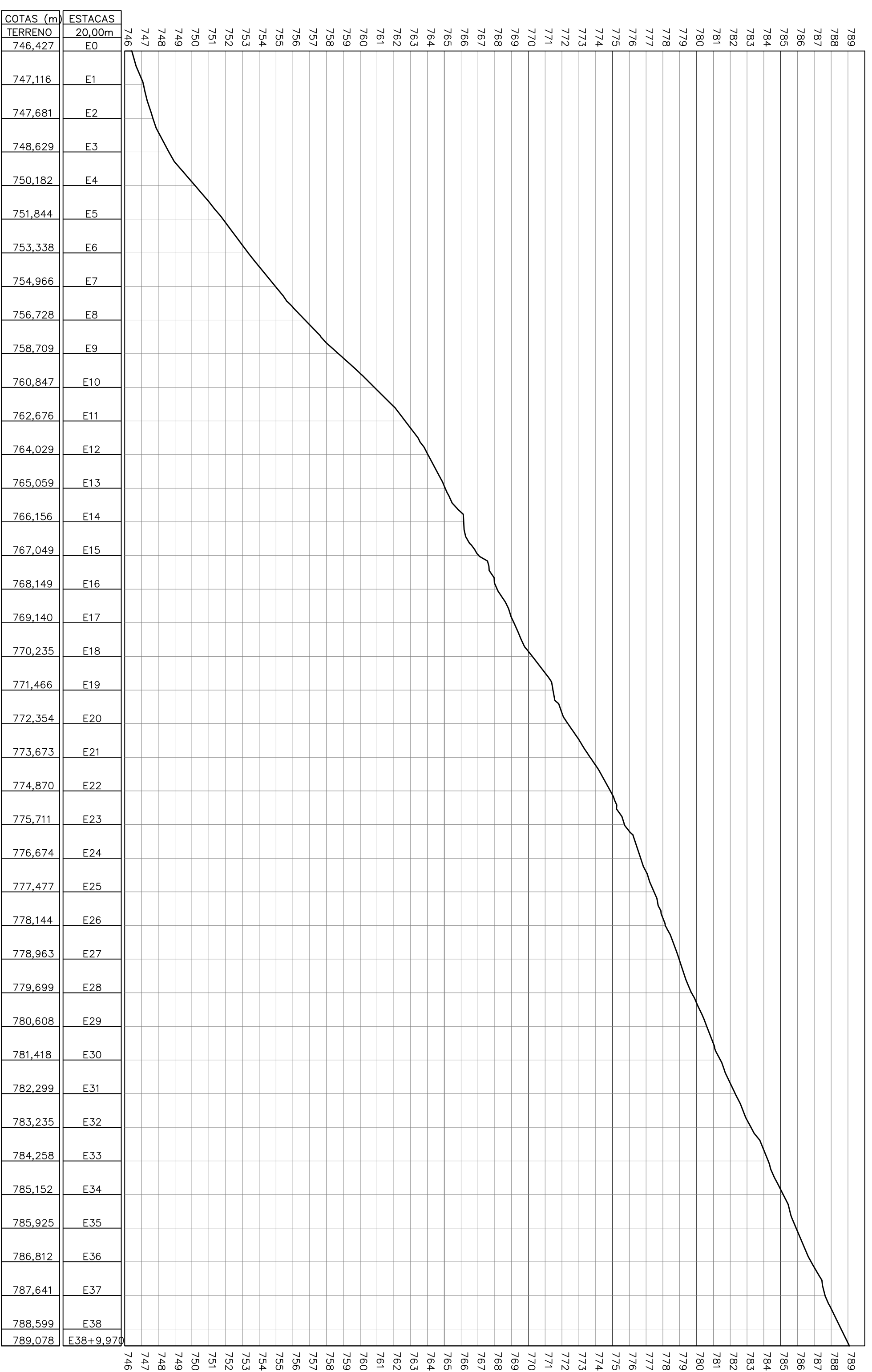
PERFIL ESC.: H=1:2000 V=1:200
