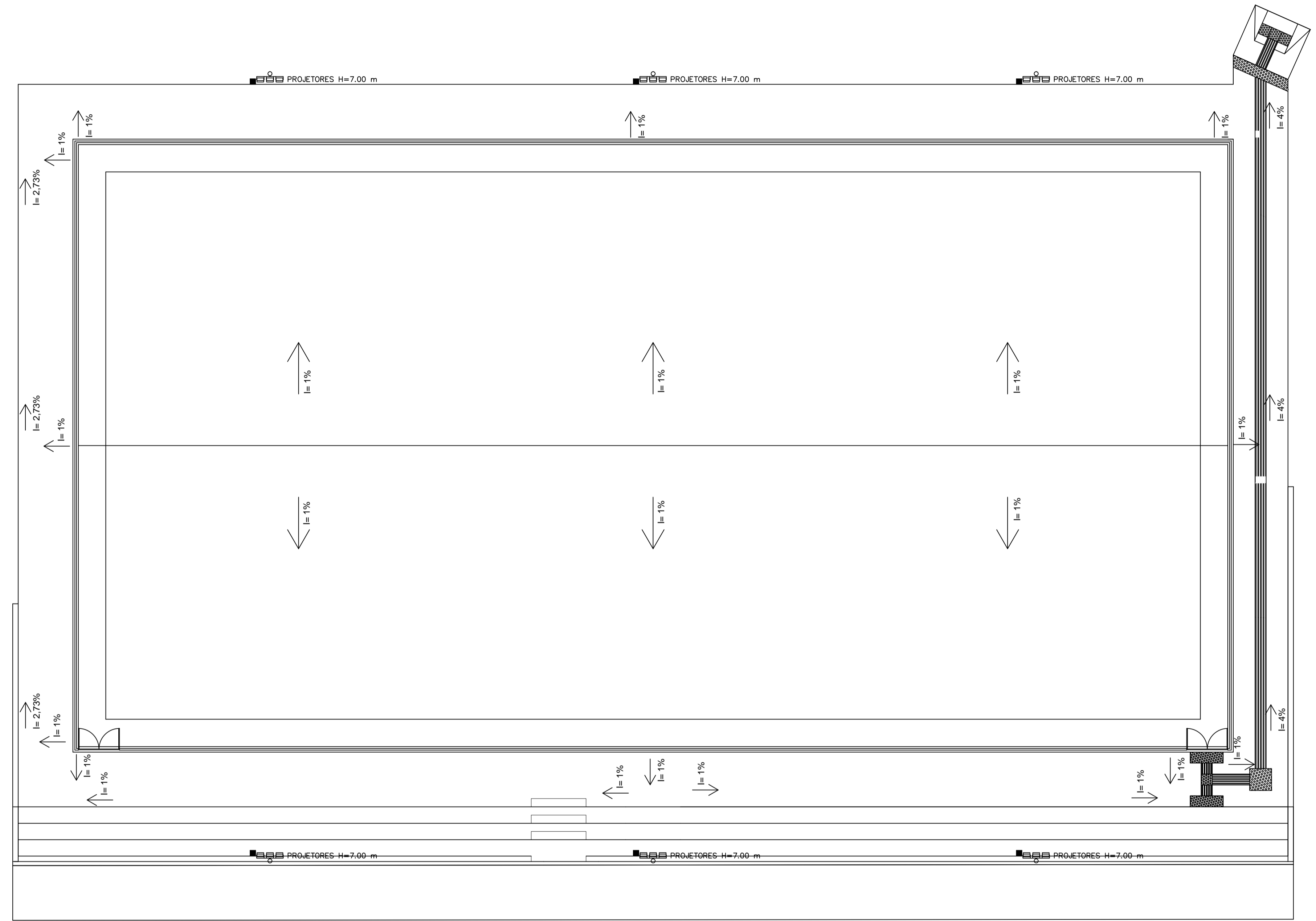
DRENAGEM ESCALA 1:100
