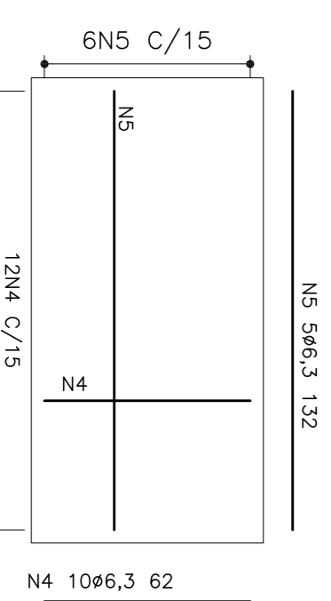
PLANTA ESC.: 1:20
