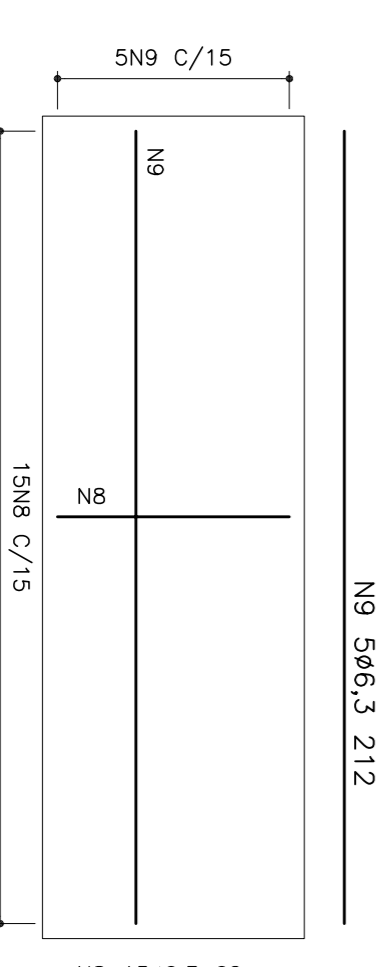
PLANTA ESC.: 1:20
