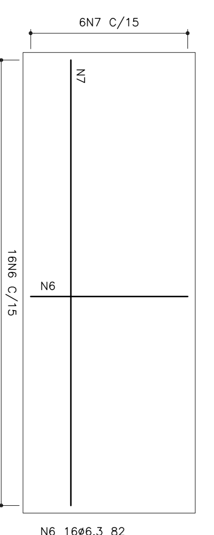
PLANTA ESC.: 1:20
